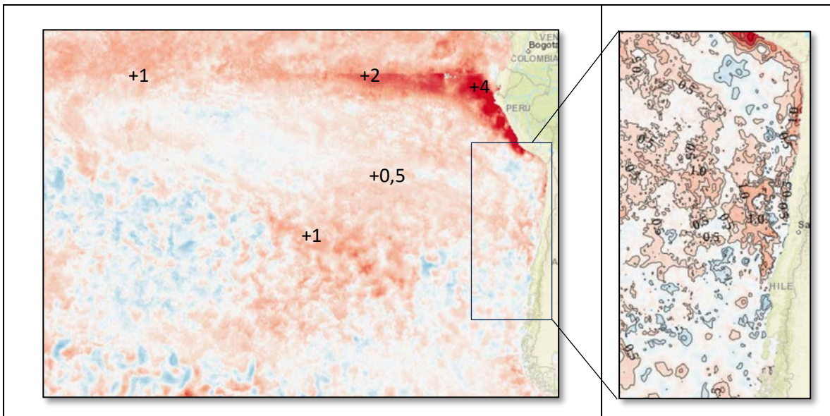
Figura 3. ATSM del océano Pacífico - costa sudamericana el 27 de mayo de 2026. La información de la ATSM fue extraída del producto MUR, calculado en base a la climatología de TSM satelital del periodo 2002 - 2026, provenientes de la plataforma S.A.P.O. IFOP (Chile).
